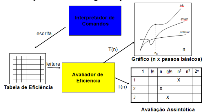
Figura 2. Arquitetura do Componente Avaliador de Eficiência
